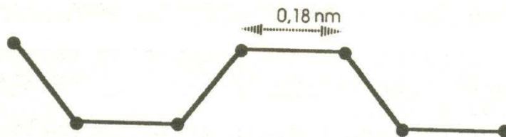
Figure IV-2- Structure unidimensionnelle du soufre « mou »
