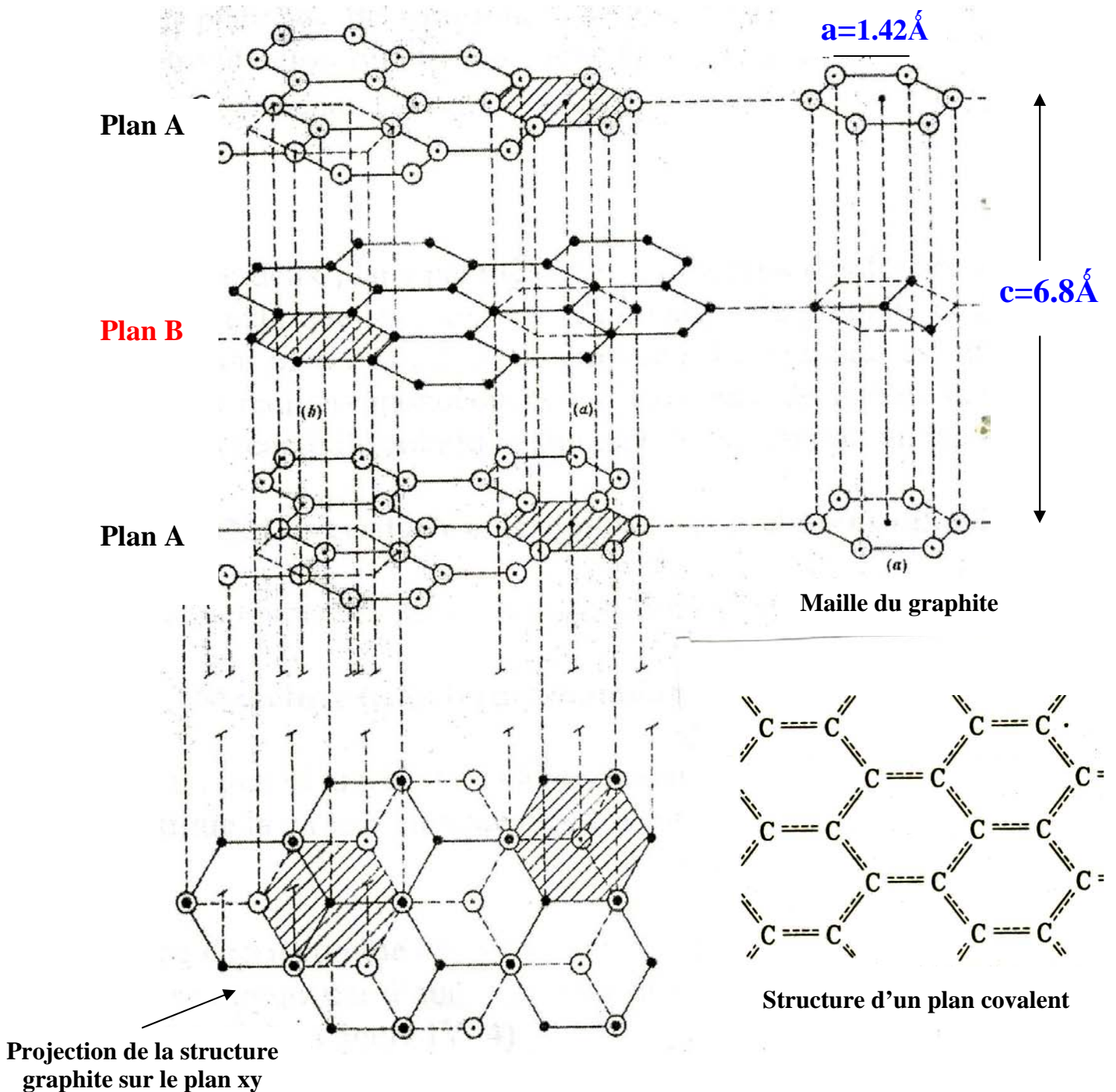
Figure IV-3- Réseau du carbone graphite
