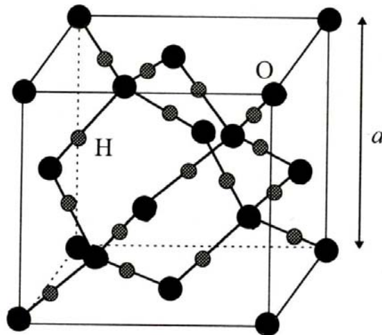
Fig. IV-5- Structure de la variété cubique de H 2 O
