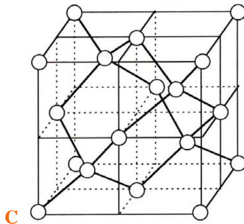
Figure IV-4- La maille élémentaire du diamant
