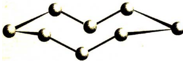
Figure IV-1- Molécule du soufre \text{S}_8
